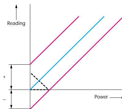
Fig. 42: Zero offset
